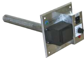
Aircode™ IDAC-100 Placering: Ventilationssystem Energiförbrukning: 35W Vikt: 2 KG Mått: L: 21 CM B: 30 CM H: 64 CM
